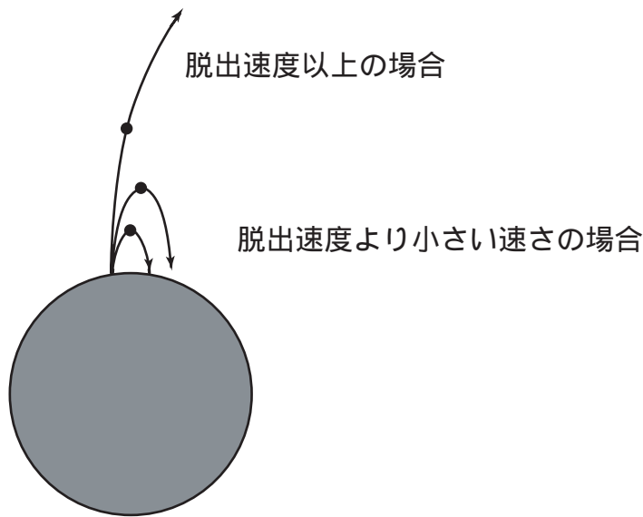
図 2: 脱出速度
