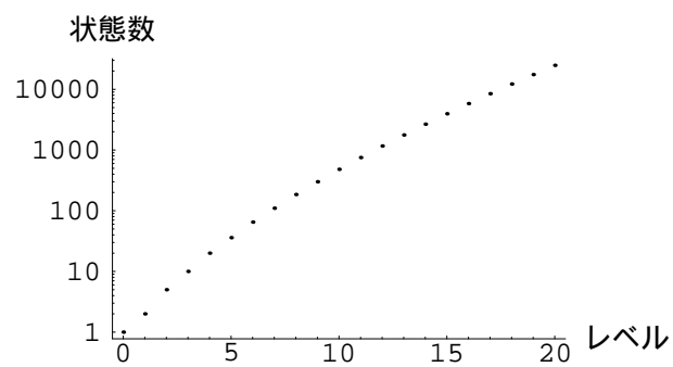
図 13: スtringの状態数が増大する様子 (4次元での端のあるStringの場合)。Y軸は対数目盛であることに注意。グラフより状態数は指数関数的に増大することがわかる。
